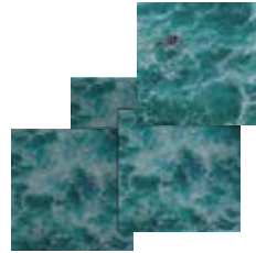
Azores SQR
